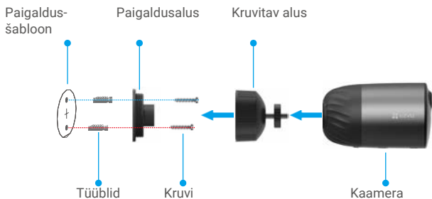
Joonis 1 Keeratava alusega paigaldamine
