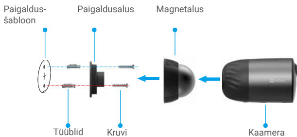
Joonis 1 Magnetialusega paigaldamine
