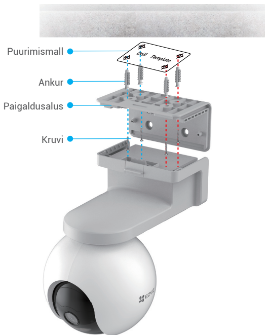
Joonis 1 Lakke kinnitamine
